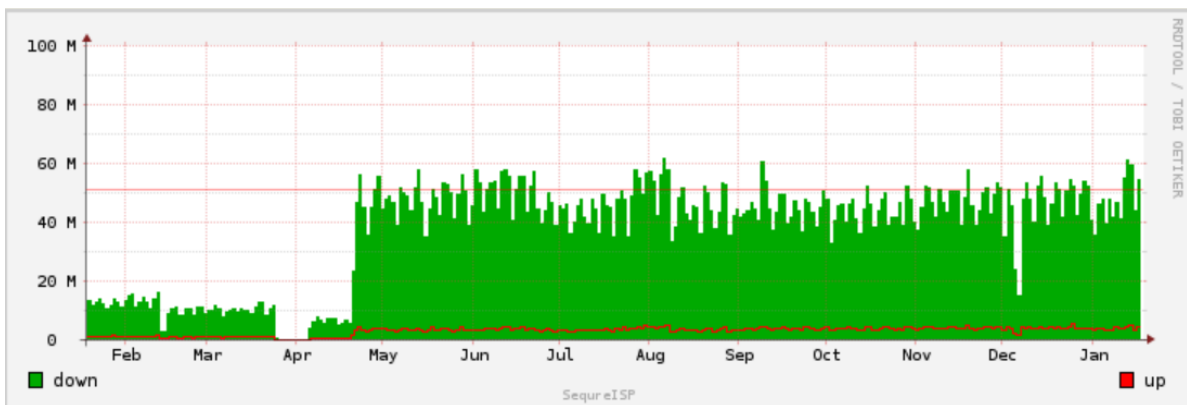
Gráfico 5. Comportamiento de Canal 5 Fibra óptica Corporativo SERKOI, durante el año 2017.
